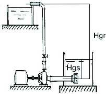
Figura 3.10 - CMB afogado
