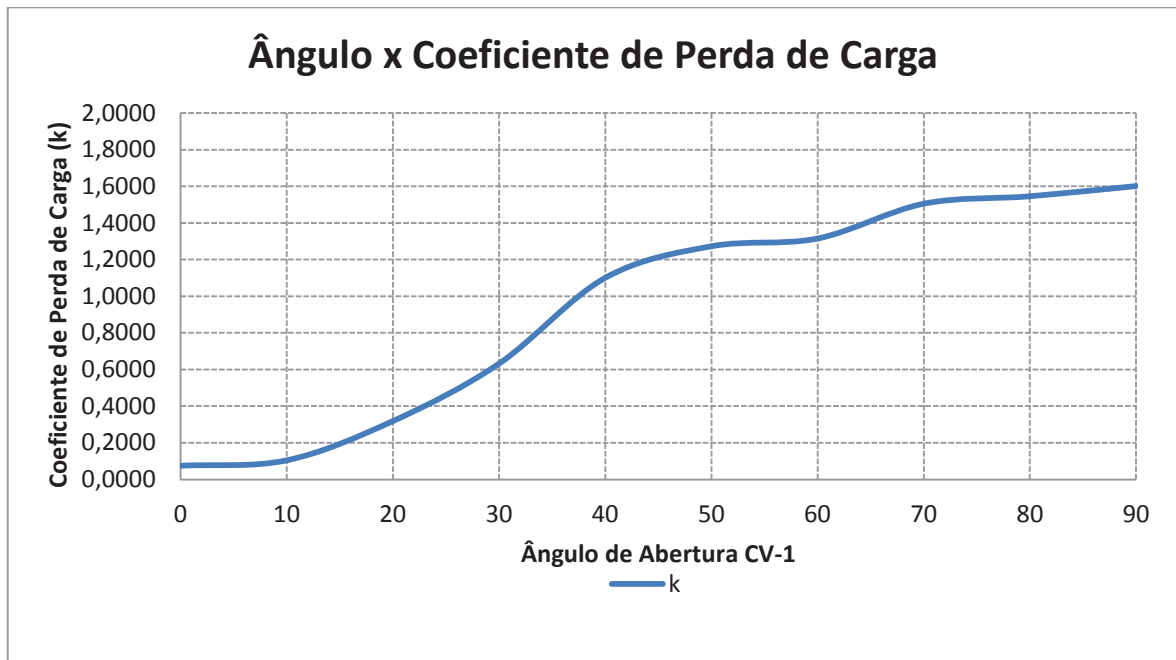
Gráfico 4.3 - Relação entre o ângulo de abertura da CV-1 com o coeficiente de perda de carga ( k )
