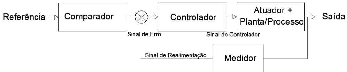
Figura 3.4 - Componentes de um sistema de controle
