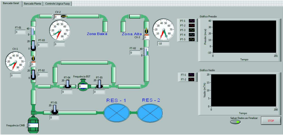
Figura A.8.1 – Interface de acionamento da bancada
