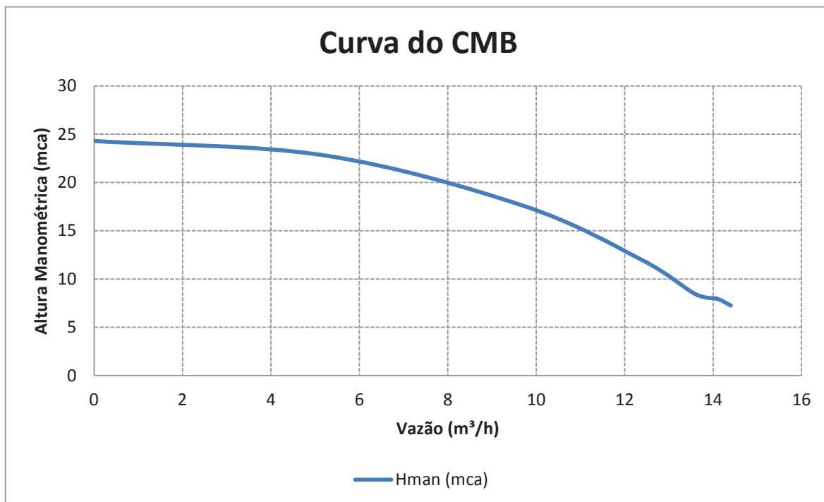
Gráfico 4.4 - Curva do CMB
