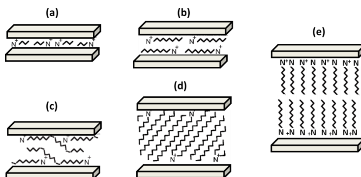
Figura 2.9 - Proposta para estruturas formadas por cátions de amônio intercalados em magadeíta em diferentes disposições: (a) monocamada, (b) bicamada, (c) pseudo-tricamada e (d,e) tipo parafina
