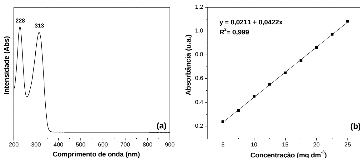
Figura 4.3 – (a) Espectro de absorção molecular da ranitidina a 15 mg dm -3 e (b) curva de calibração.
