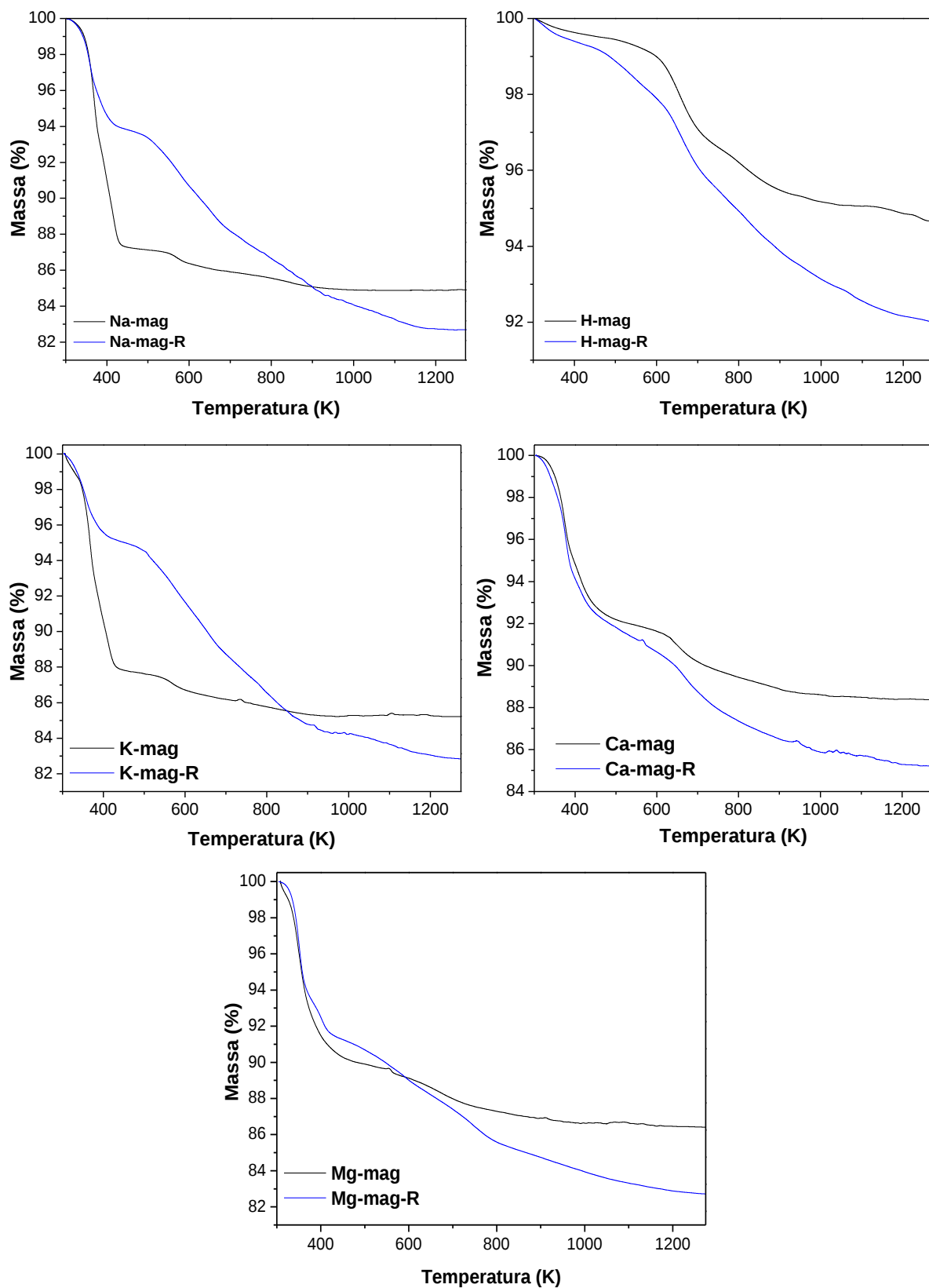
Figura 4.16 - Curvas termogravimétricas (TG) para as matrizes antes e após interação com a ranitidina.
