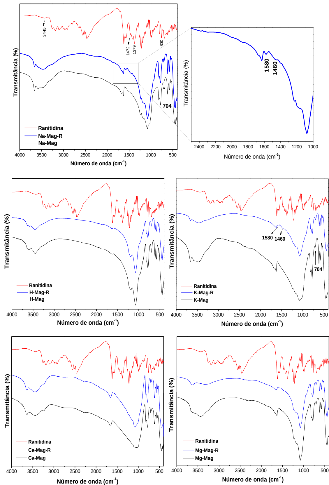
Figura 4.15 - Espectros de infravermelho das matrizes iniciais, híbridos magadeíta-fármaco e da ranitidina.
