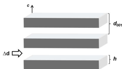
Figura 2.1 - Representação esquemática do empilhamento das camadas de um sólido lamelar ao longo do eixo c, mostrando o espaçamento basal ( d_{001} ), altura da camada ( h ) e espaço interlamelar ( \Delta d ).
