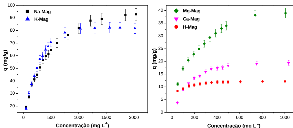
Figura 4.10 – Efeito da concentração na adsorção de ranitidina em Na-, H-, K-, Ca- e Mg- magadeíta
