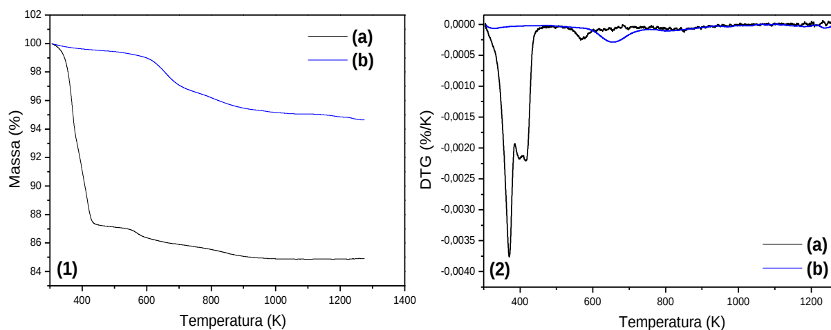
Figura 3.5 - Curvas (1) termogravimétricas e (2) suas derivadas (DTG) para (a) Na-magadeíta e (b) H-magadeíta.
