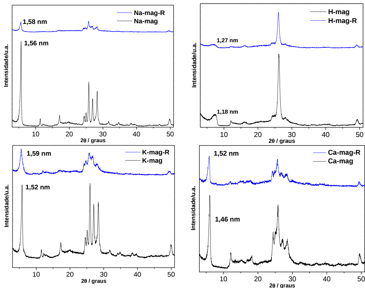
Figura 4.13 – Difratomogramas de raios X dos sólidos antes e após interação com a ranitidina.
