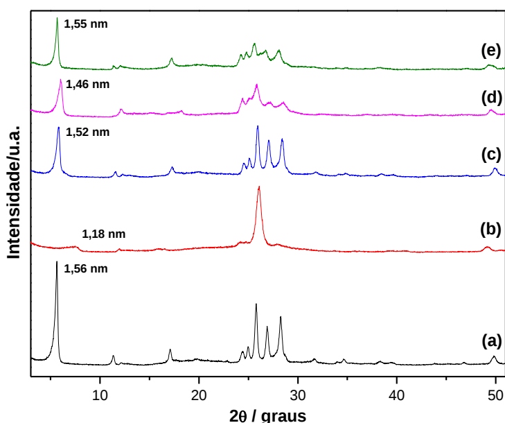
Figura 4.5 – Difratogramas de raios X da (a) Na-mag, (b) H-mag, (c) K-mag, (d) Ca-mag e (e) Mg-mag
