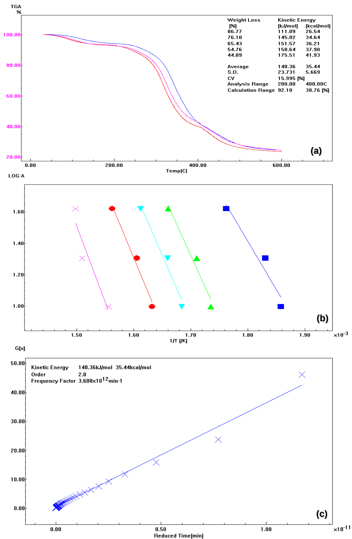
Figura A4. Curvas TG para filmes de GX/PVA/AC (20%) nas diferentes taxas de aquecimento (10, 20 e 40°C/min) (a) , gráfico \log \beta versus 1/T para GX (b) e o gráfico da função G(X) pelo tempo reduzido (c) .
