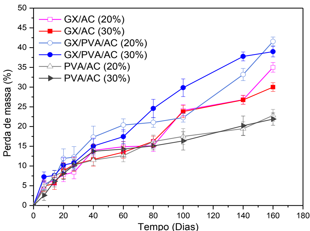
Figura 35. Biodegradação em solo (perda de massa) das composições reticuladas com 20 e 30% AC em um período de 160 dias.
