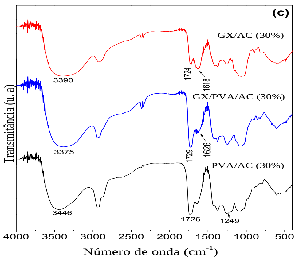
Figura 24. Espectros de infravermelho obtidos para os filmes formados por GX e PVA não reticulados (a) , reticulados com 20 (b) e 30% (c) de ácido cítrico.
