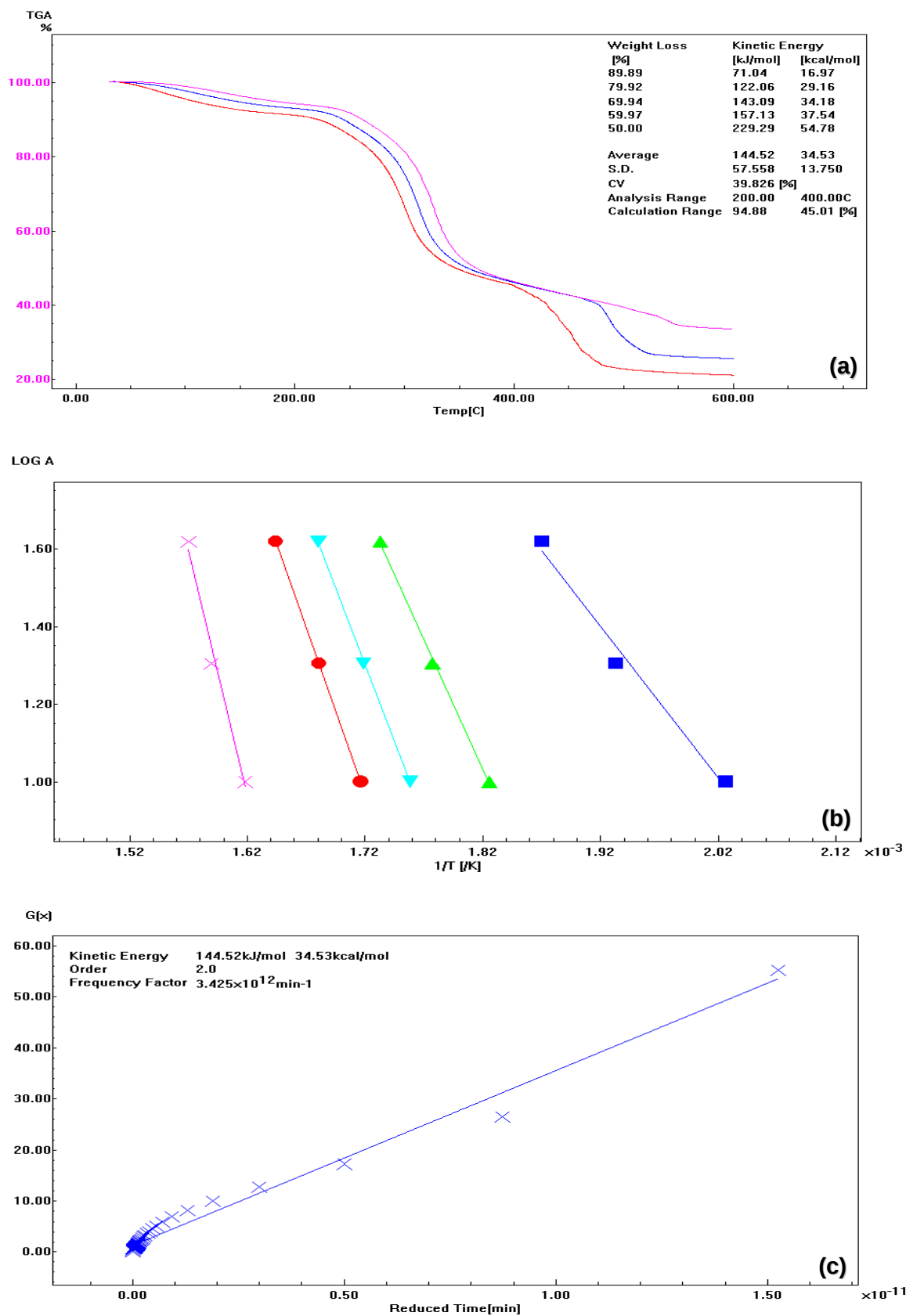
Figura A1. Curvas TG para filmes de GX/AC (20%) nas diferentes taxas de aquecimento (10, 20 e 40°C/min) (a), gráfico \log \beta versus 1/T para GX (b) e o gráfico da função G(X) pelo tempo reduzido (c).
