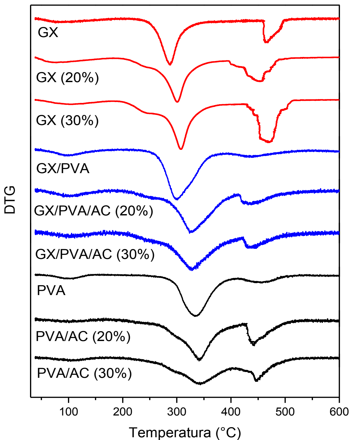
Figura 32. DTG obtidas para as diferentes composições de filmes poliméricos analisados sob atmosfera inerte, no intervalo de 25-600°C.
