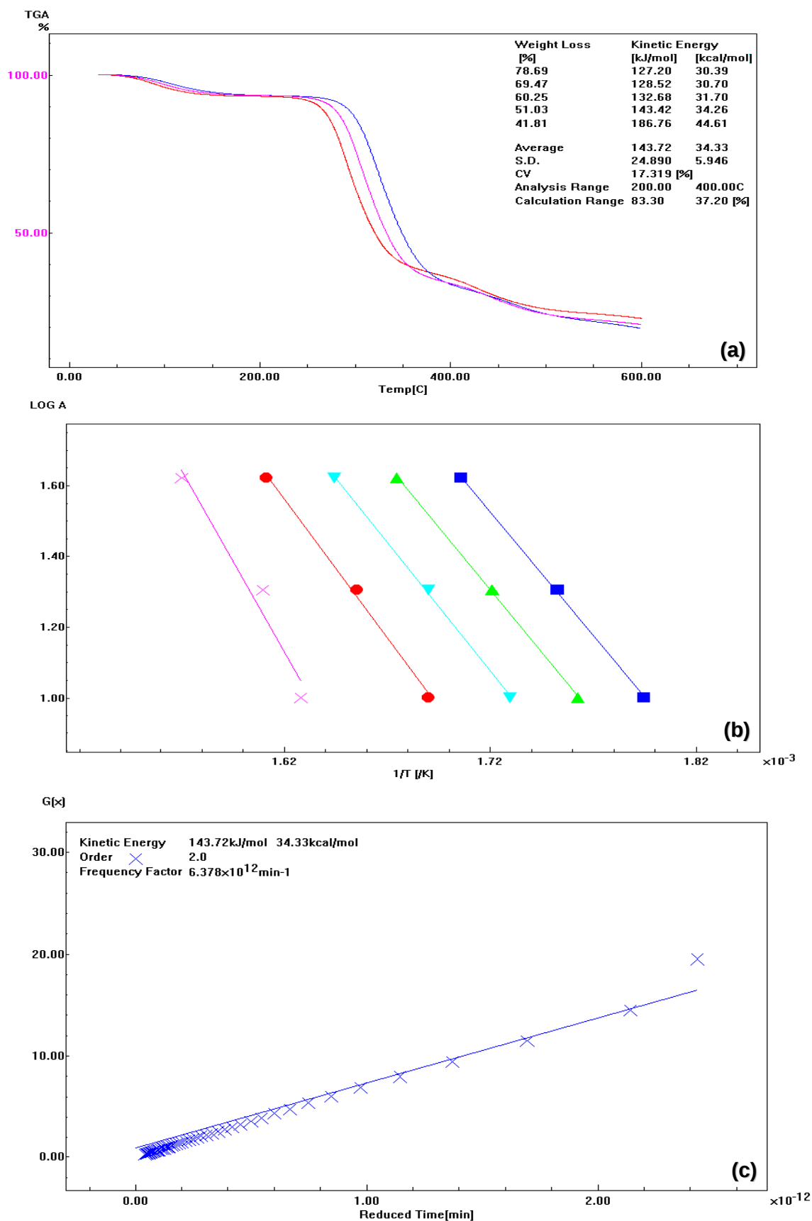
Figura A3. Curvas TG para filmes de GX/PVA nas diferentes taxas de aquecimento (10, 20 e 40 °C/min) (a) , gráfico \log \beta versus 1/T para GX (b) e o gráfico da função G(X) pelo tempo reduzido (c) .
