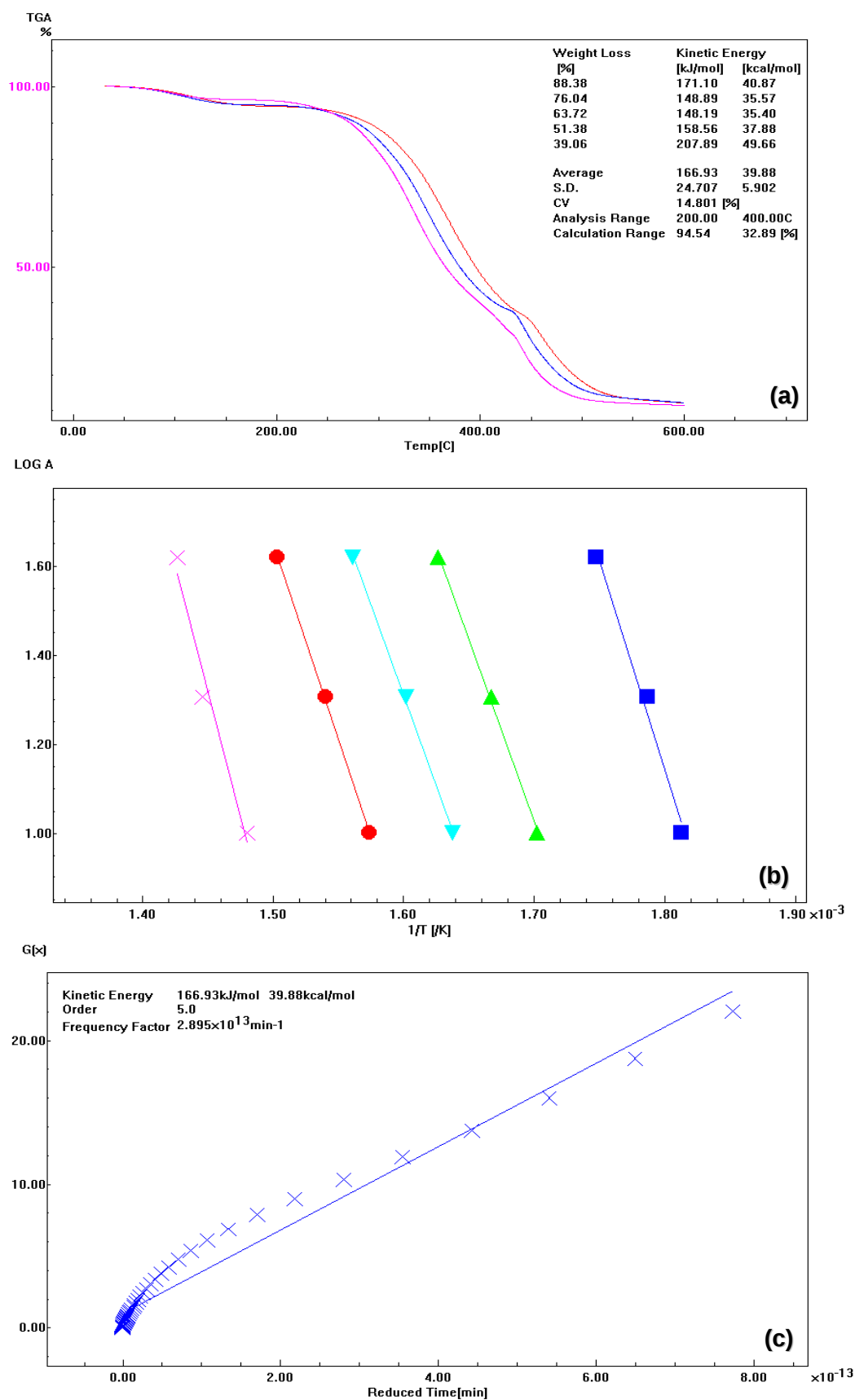
Figura A8. Curvas TG para filmes de PVA/AC (30%) nas diferentes taxas de aquecimento (10, 20 e 40°C/min) (a) , gráfico \log \beta versus 1/T para GX (b) e o gráfico da função G(X) pelo tempo reduzido (c) .
