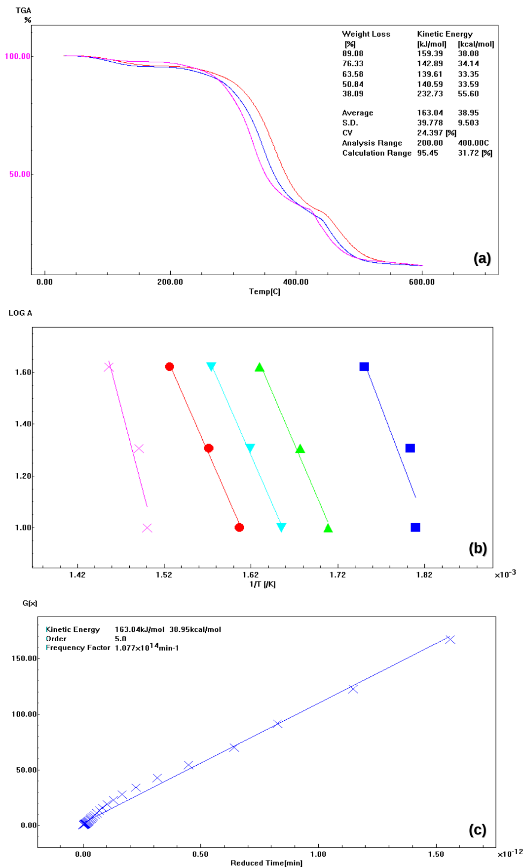
Figura A7. Curvas TG para filmes de PVA/AC (20%) nas diferentes taxas de aquecimento (10, 20 e 40 °C/min) (a) , gráfico log \beta versus 1/T para GX (b) e o gráfico da função G(X) pelo tempo reduzido (c) .
