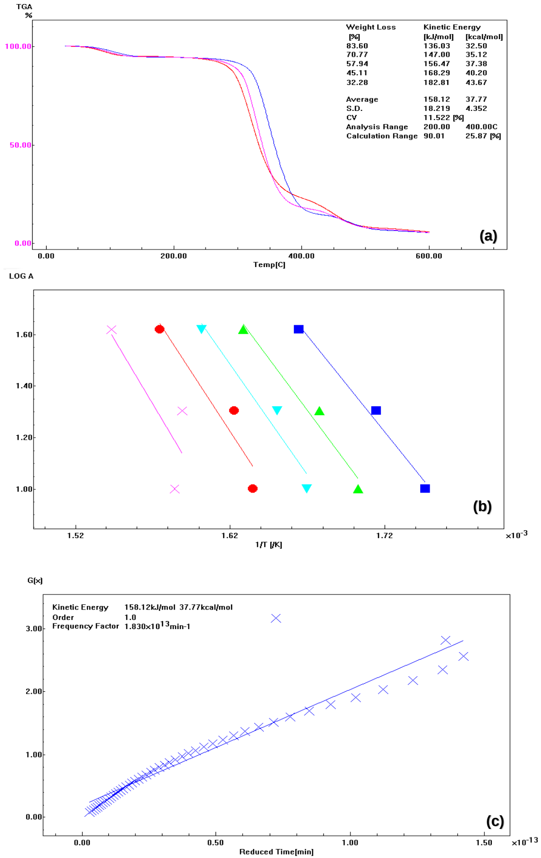
Figura A6. Curvas TG para filmes de PVA nas diferentes taxas de aquecimento (10, 20 e 40°C/min) (a) , gráfico \log \beta versus 1/T para GX (b) e o gráfico da função G(X) pelo tempo reduzido (c) .
