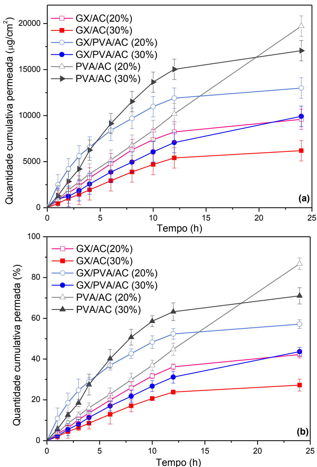
Figura 38. Perfis de liberação/permeação do paracetamol a partir dos filmes de GX/PVA reticulado com ácido cítrico. Gráfico da quantidade cumulativa de paracetamol liberado ( Q , \mu\text{g cm}^{-2} ) pelo tempo (h) (a) . Gráfico da percentagem da quantidade cumulativa permeada (%) em relação ao tempo (h) (b) . As barras de erros indicam a variabilidade a partir de três replicatas ( n=3 ).
