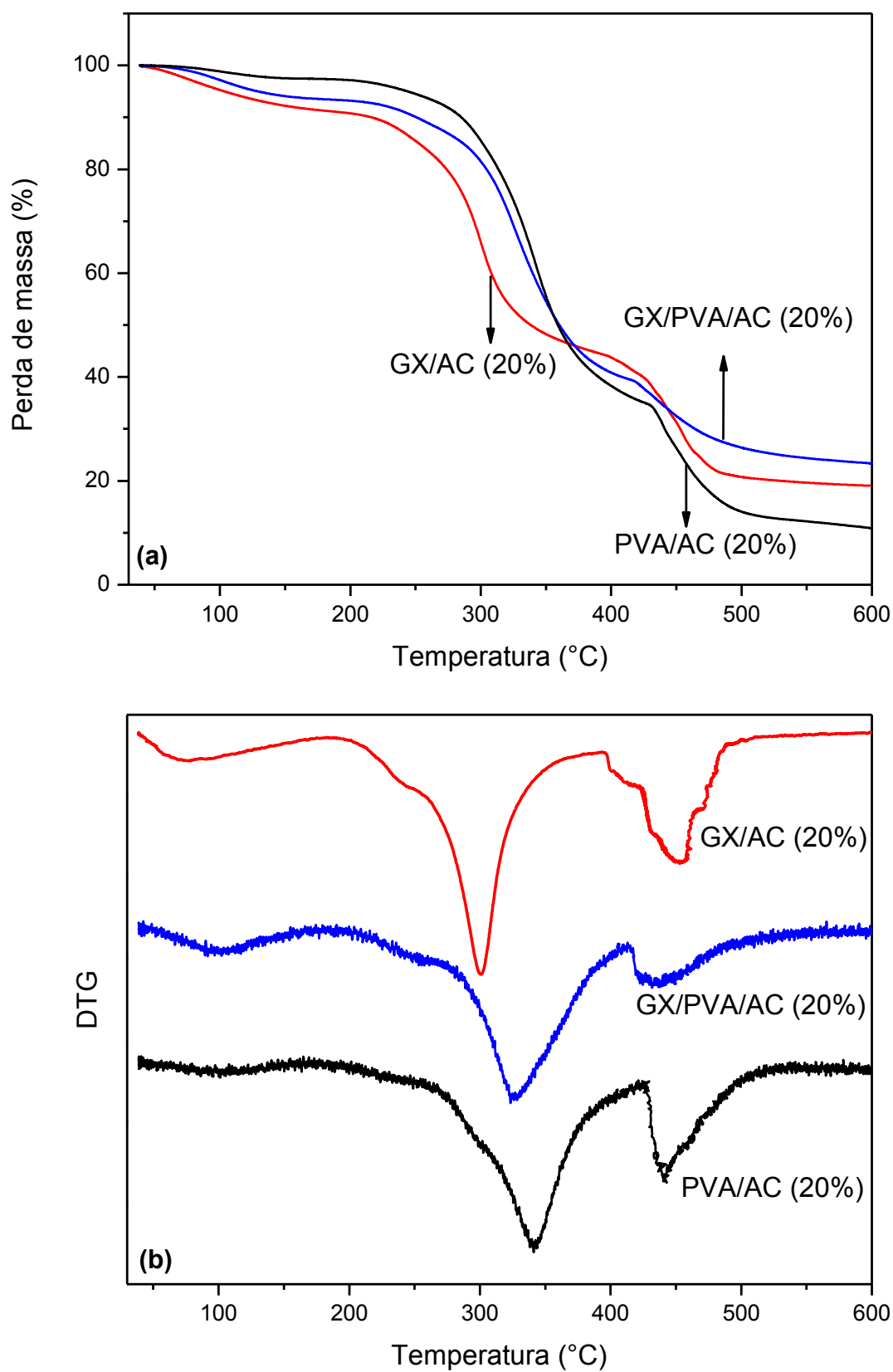
Figura 30. Curvas termogravimétricas (a) e suas derivadas (DTG) (b) obtidas para os filmes de GX e PVA reticulados com 20% de AC analisadas sob atmosfera inerte, no intervalo de 25-600°C.
