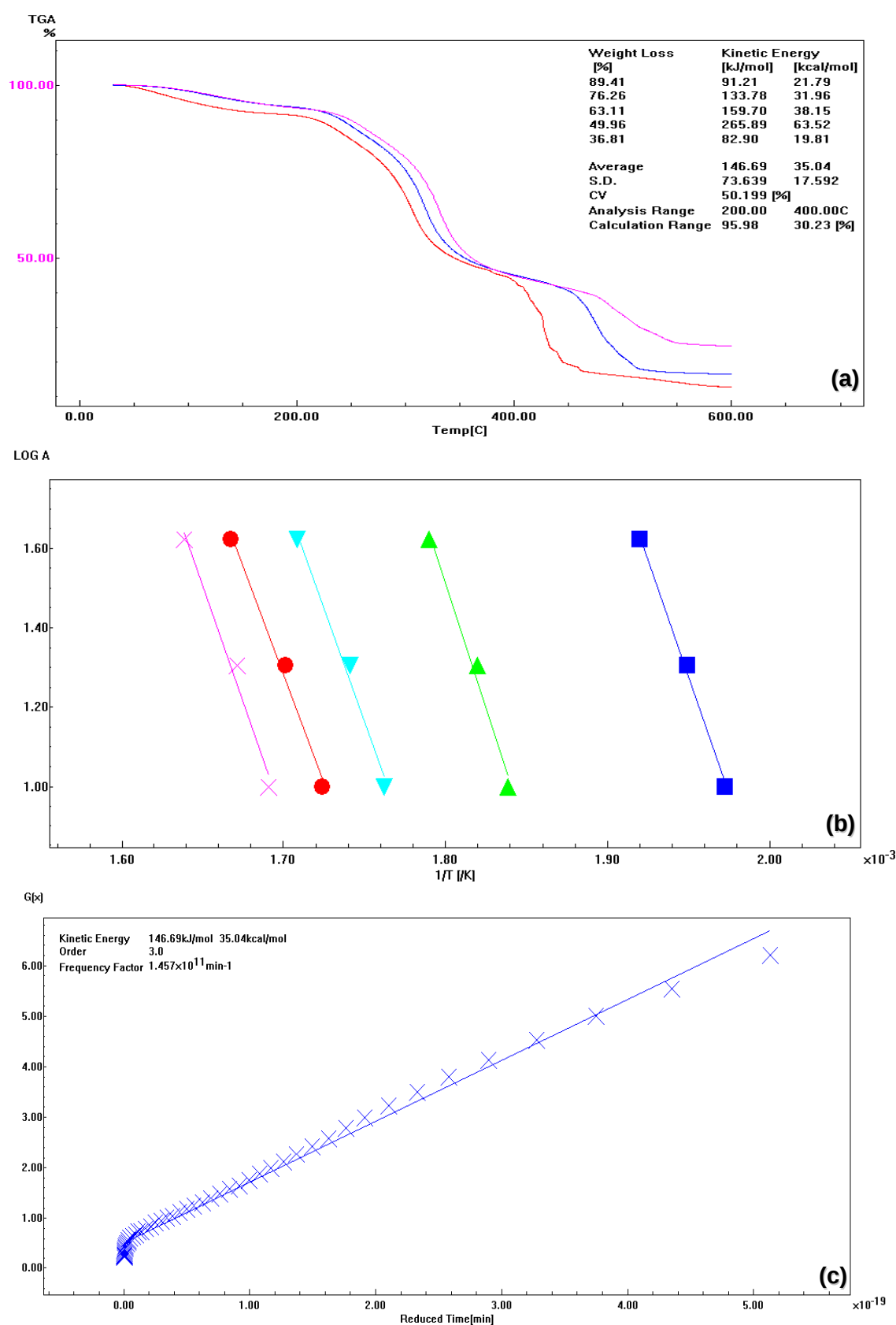
Figura A2. Curvas TG para filmes de GX/AC (30%) nas diferentes taxas de aquecimento (10, 20 e 40°C/min) (a) , gráfico log \beta versus 1/T para GX (b) e o gráfico da função G(X) pelo tempo reduzido (c) .
