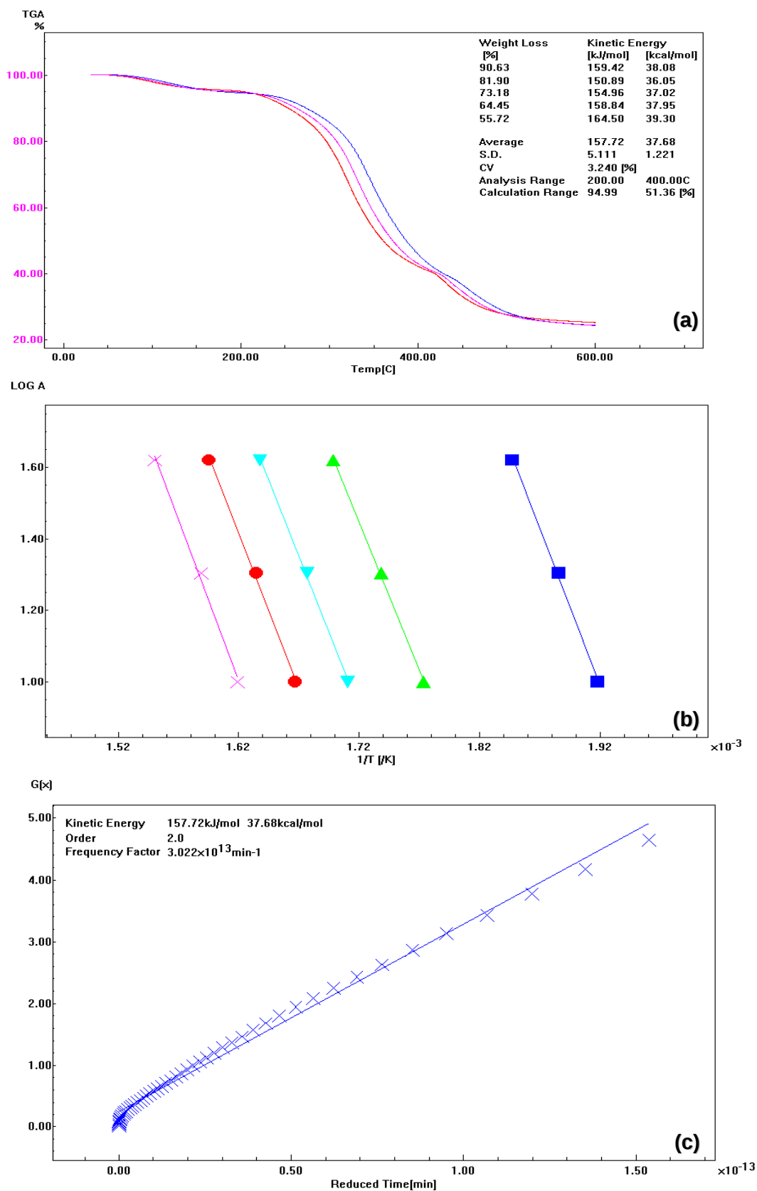
Figura A5. Curvas TG para filmes de GX/PVA/AC (30%) nas diferentes taxas de aquecimento (10, 20 e 40°C/min) (a) , gráfico \log \beta versus 1/T para GX (b) e o gráfico da função G(X) pelo tempo reduzido (c) .
