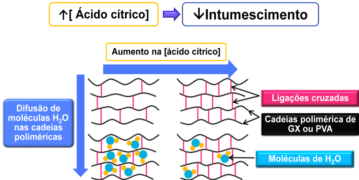
Figura 28. Intumescimento das cadeias poliméricas. Relação da concentração de AC com o intumescimento (Fonte: Adaptada de LEE; YEO, 2015).
