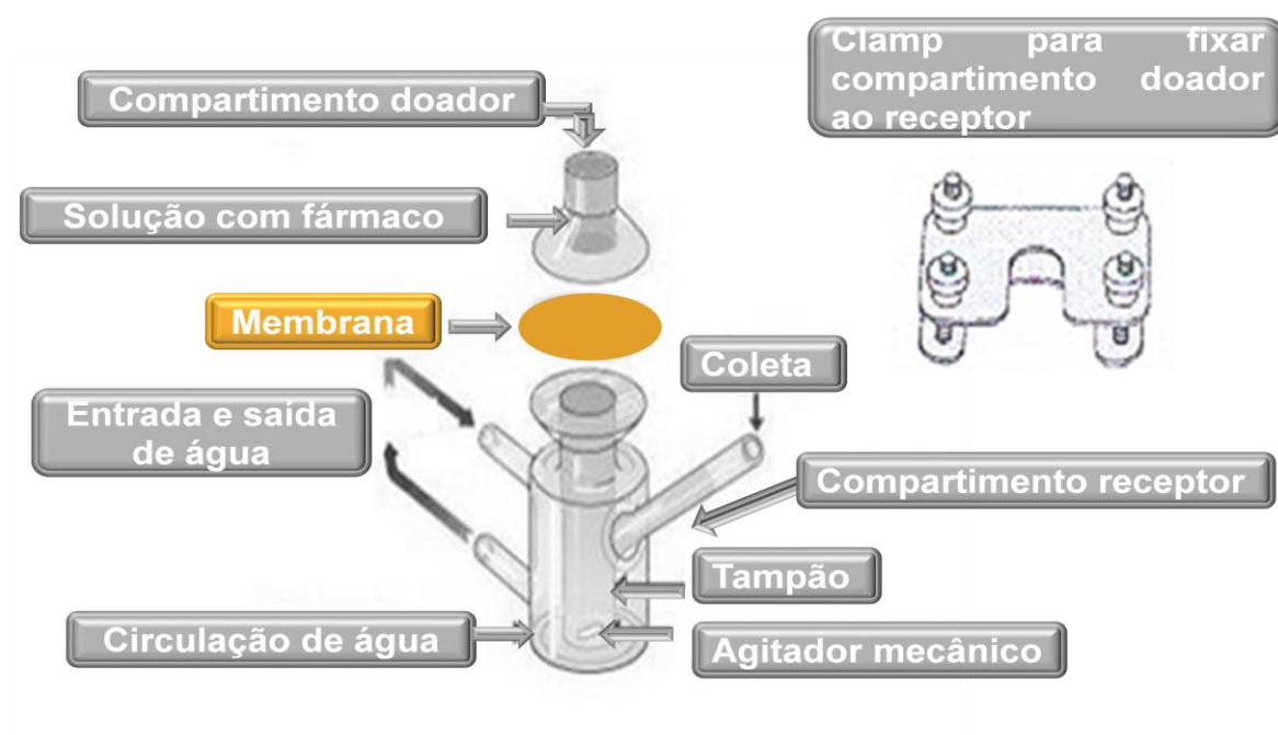
Figura 19. Representação da célula de difusão de Franz. (Fonte: Adaptada de SILVA et al. , 2008).
