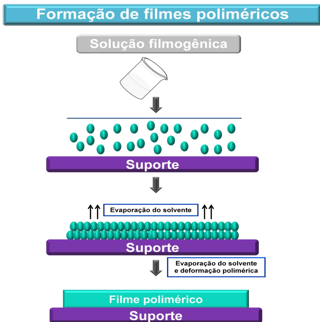
Figura 16. Processo de formação de filmes poliméricos pelo método de evaporação do solvente (Fonte: Adaptado de FELTON, 2013; SIEPMANN et al. , 2008).
