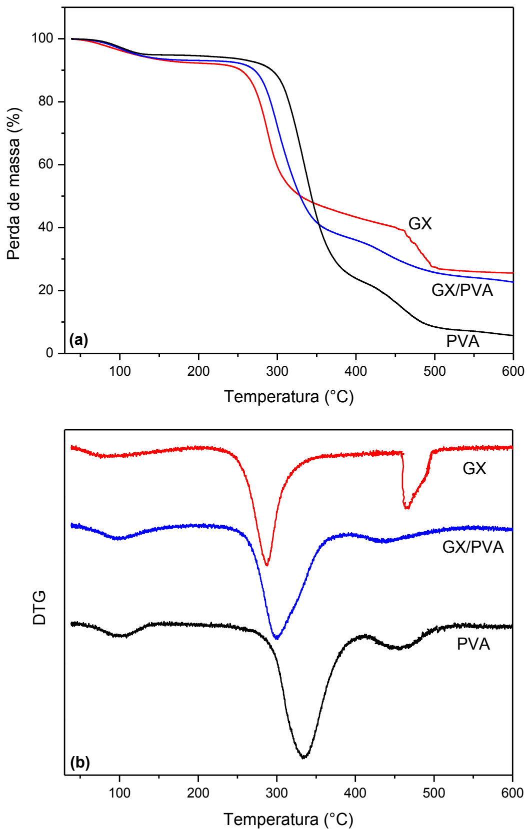
Figura 29. Curvas termogravimétricas (a) e suas derivadas (DTG) (b) obtidas para os filmes de GX e PVA não reticulados analisadas sob atmosfera inerte, no intervalo de 25-600°C.
