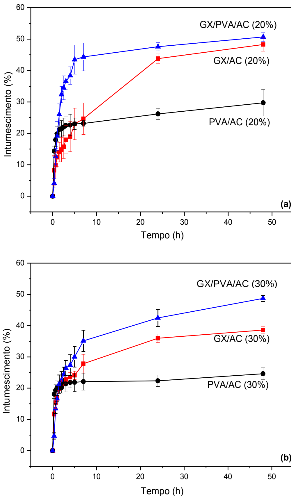
Figura 27. Cinética de intumescimento dos filmes constituídos por GX/PVA reticulados com 20 (a) e 30% (b) de ácido cítrico em diferentes tempos de imersão em água durante um período de 48 h.
