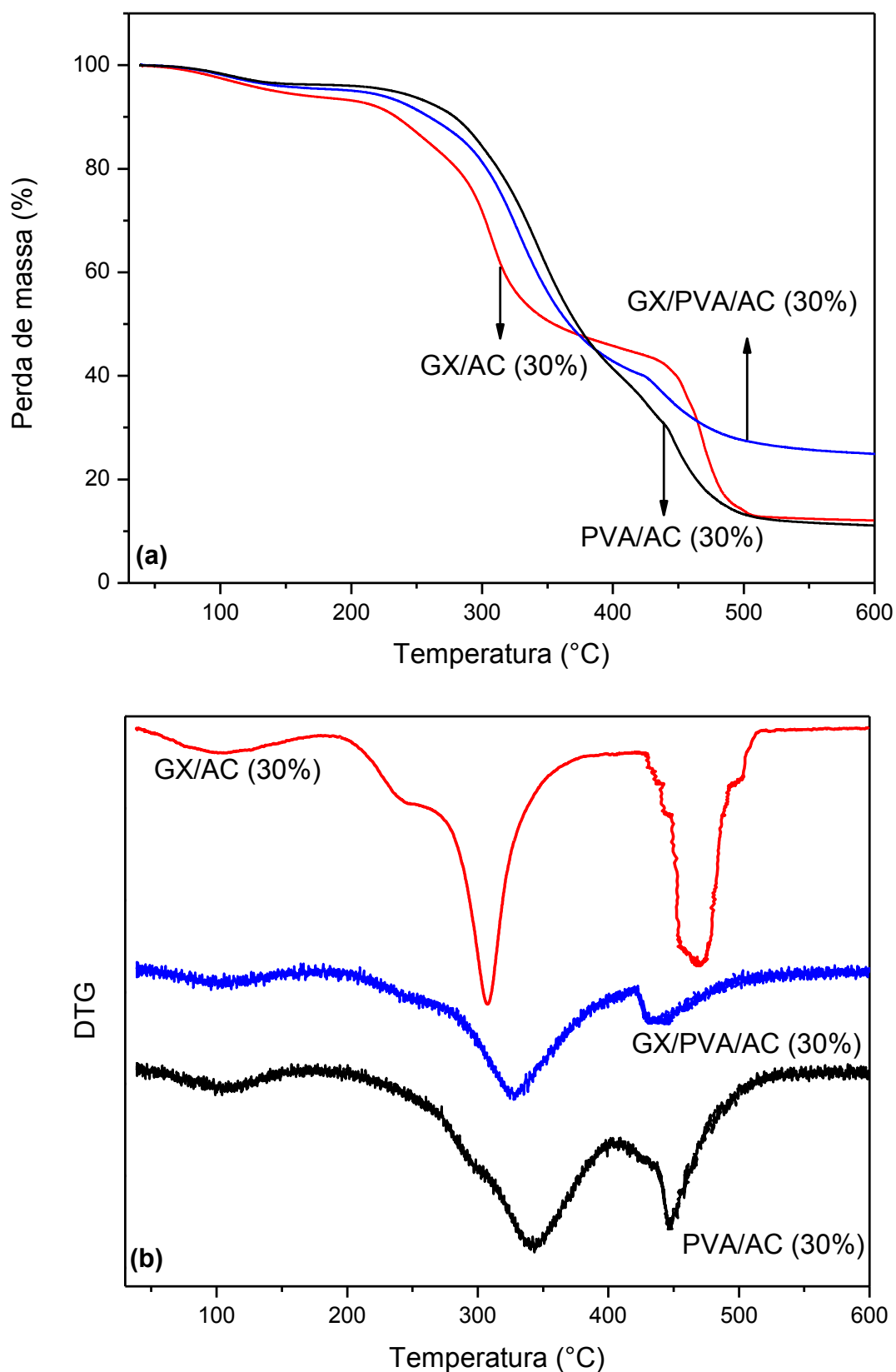
Figura 31. Curvas termogravimétricas (a) e suas derivadas (DTG) (b) obtidas para os filmes de GX e PVA reticulados com 30% de AC analisadas sob atmosfera inerte, no intervalo de 25-600°C.
