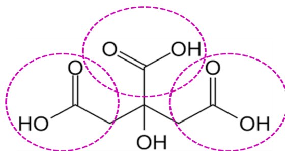
Estrutura multicarboxílica
