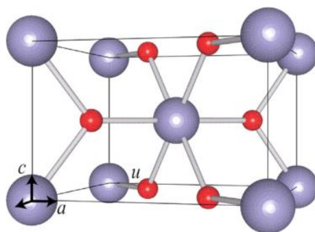
Figura 4. Estrutura cristalina do \text{SnO}_2 (DAS; JAYARAMAN, 2014).
