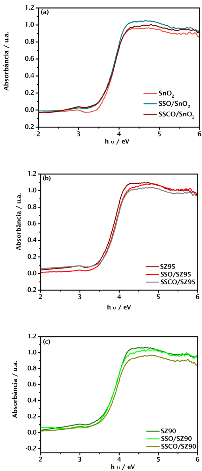
Figura 43. Espectros de absorção UV-vis das fases ativas impregnadas sobre os suportes catalíticos (a) \text{SnO}_2 ; (b) \text{SZ95} ; (c) \text{SZ90} calcinados a 800^\circ\text{C} / 4 horas.
