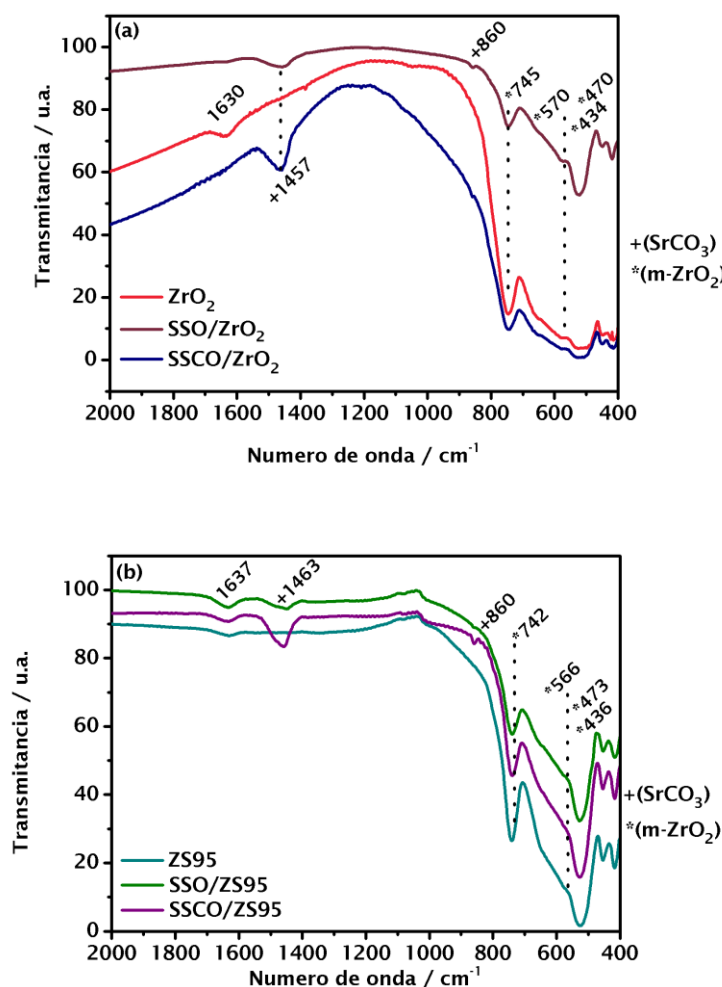
Figura 37. Espectros vibracionais na região do infravermelho das fases ativas impregnadas sobre os suportes (a) \text{ZrO}_2 e (b) ZS95, calcinados a 800^\circ\text{C} / 4 horas.
