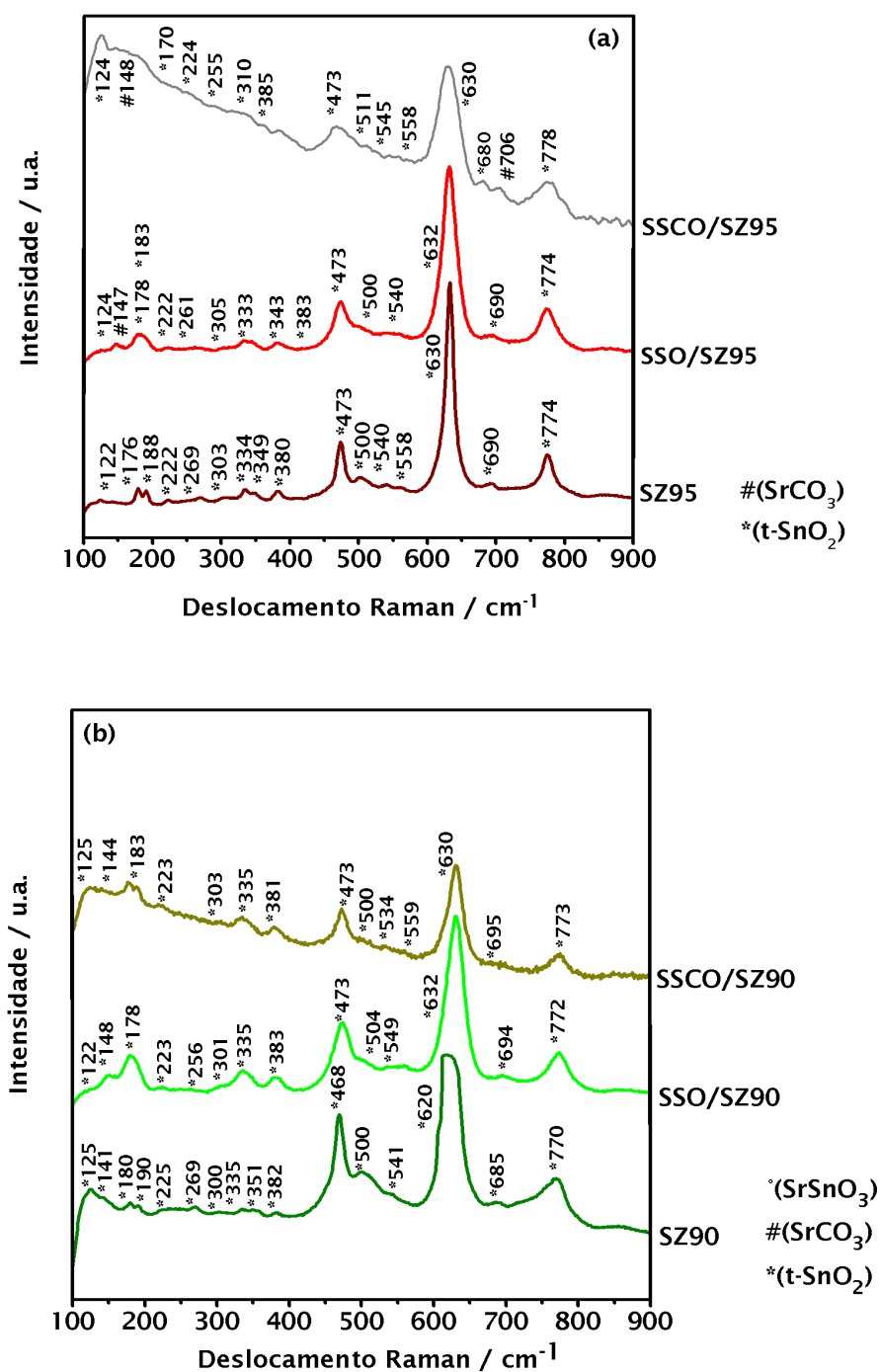
Figura 40. Espectros Raman das fases ativas impregnadas sobre os suportes catalíticos (a) SZ95 e (b) SZ90 calcinados a 800^\circ\text{C} / 4 horas.
