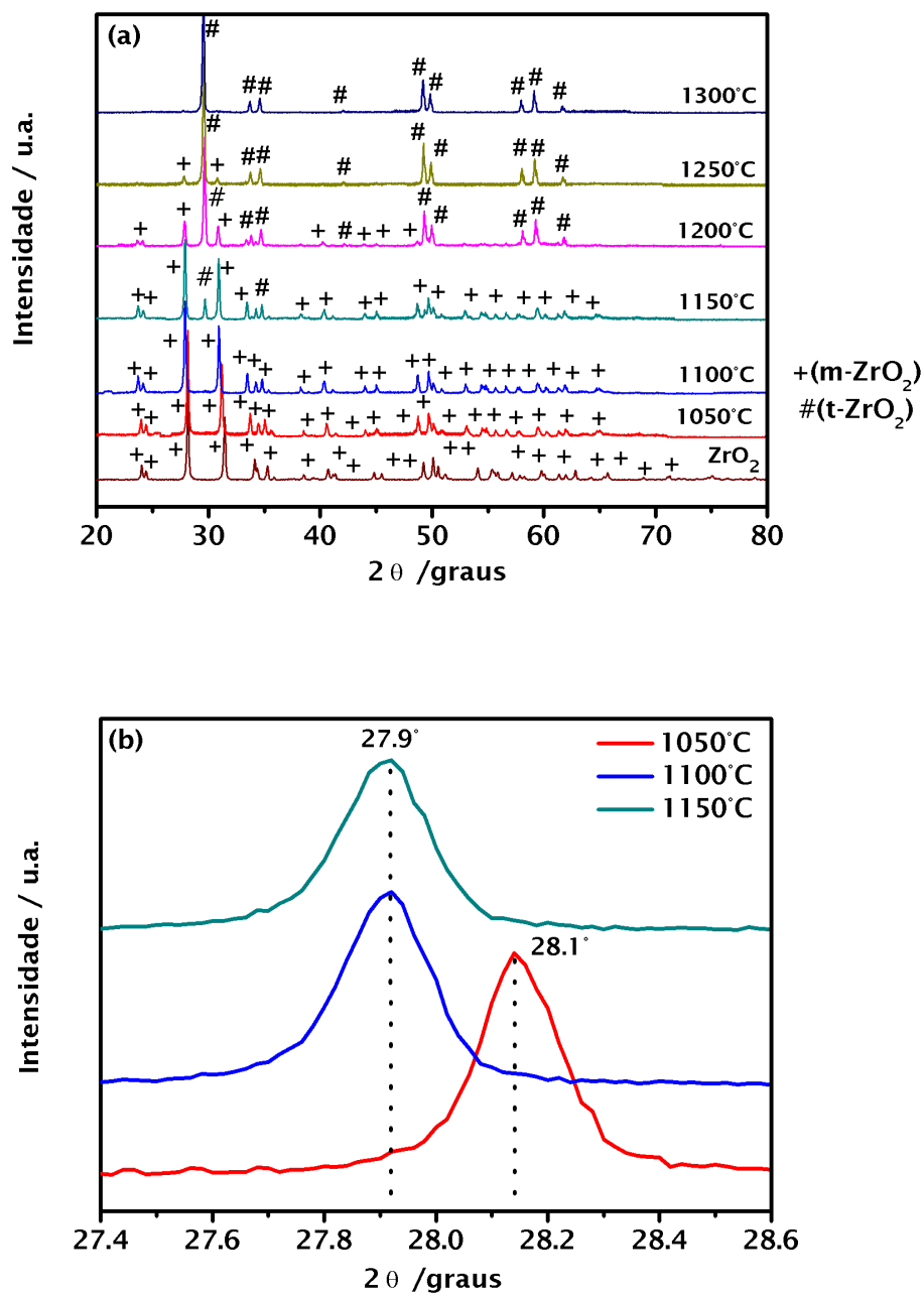
Figura 22. (a) Difratoograma de raios-X do suporte \text{ZrO}_2 obtido em câmara quente a diferentes temperaturas e (b) Deslocamento do pico em 2\theta = 28.2^\circ referente ao plano (\bar{1} 1 1) da m\text{-ZrO}_2 .
