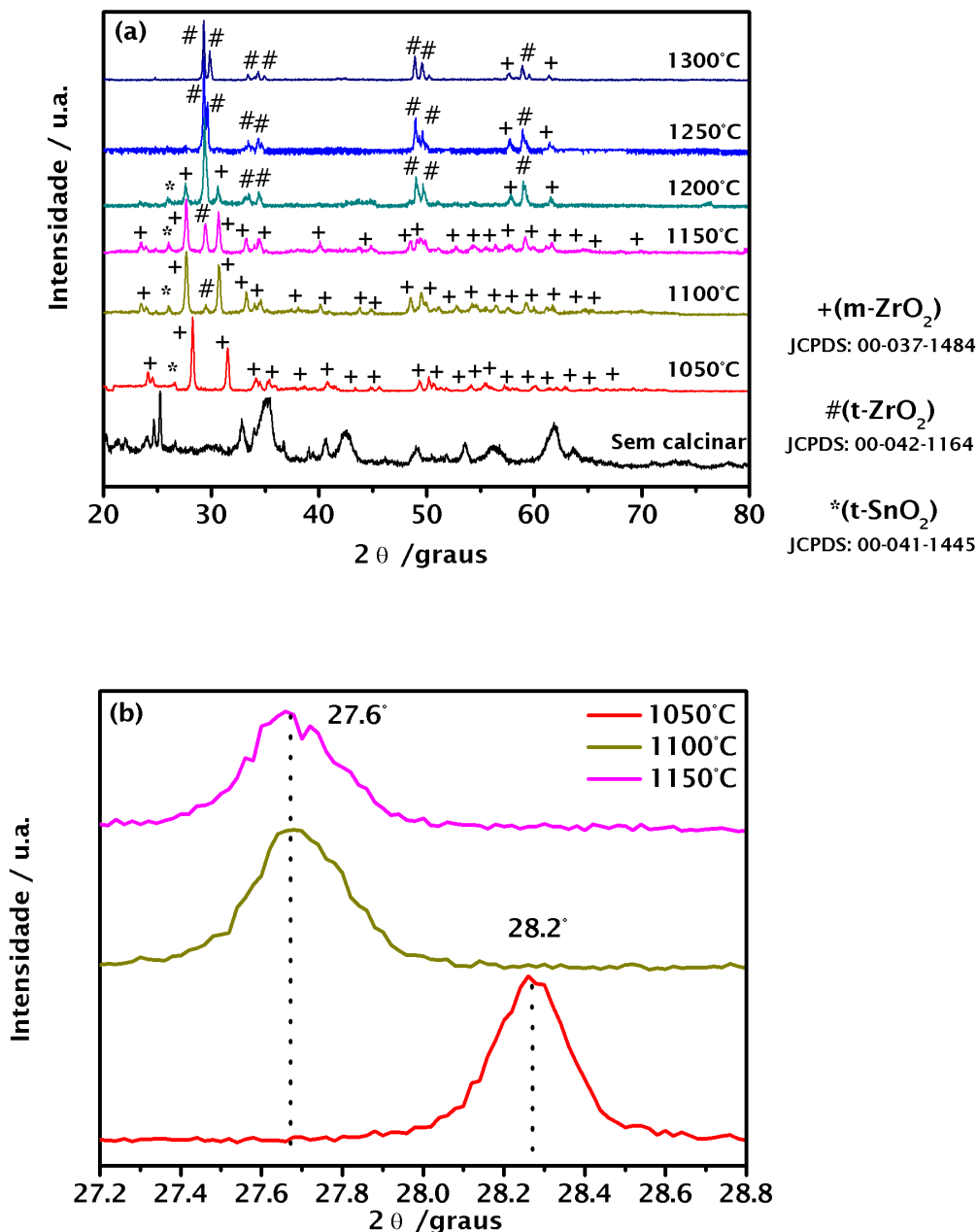
Figura 23. (a) Difratoograma de raios-X do suporte ZS95 obtido em câmara quente a diferentes temperaturas e (b) Deslocamento do pico em 2\theta = 28.2^\circ referente ao plano (\bar{1}11) da m-ZrO_2 .
