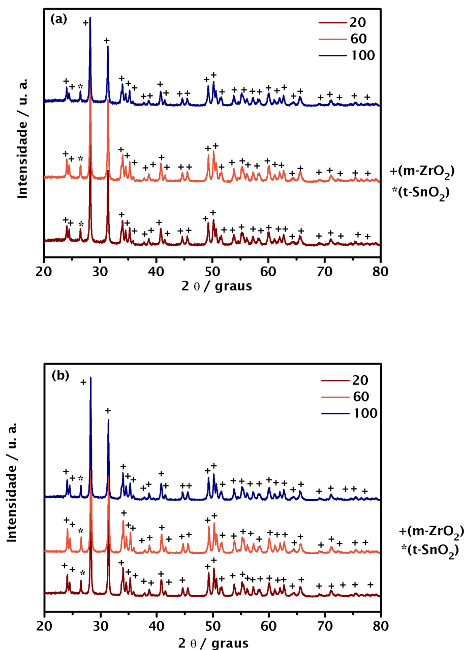
Figura 18. Difratoograma do suporte ZS90 em diferentes pressões: (a) 1300^\circ\text{C}/6 h; (b) 1300^\circ\text{C}/10 h.
