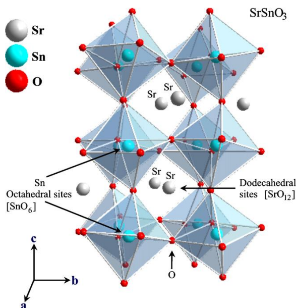
Figura 2. Modelo esquemático do \text{SrSnO}_3 de estrutura ortorrômbica ( Pbnm ) (BOHNEMANN et al., 2009).
