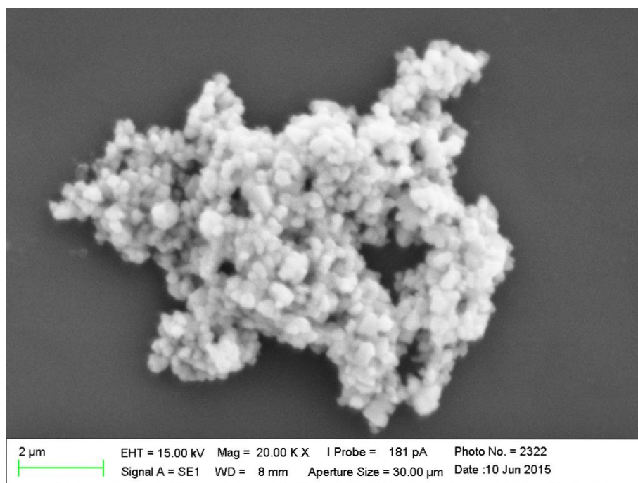
Figura 30. Micrografias do suporte comercial \text{ZrO}_2 .
