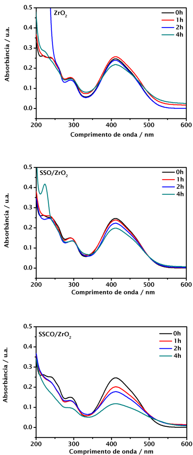
Figura 49. Espectros de UV-Vis do corante Remazol Amarelo Ouro após 1, 2 e 4 horas de irradiação UVC dos materiais impregnados sobre \text{ZrO}_2 .
