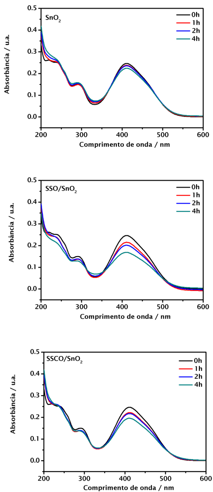
Figura 46. Espectros de UV-Vis do corante Remazol Amarelo Ouro após 1, 2 e 4 horas de irradiação UVC dos materiais impregnados sobre SnO 2 .
