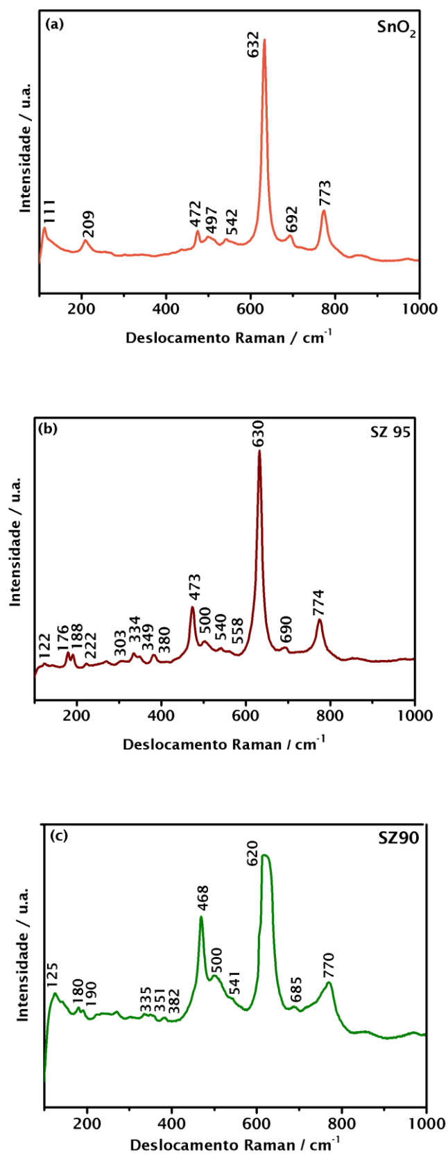
Figura 26. Espectros Raman dos suportes (a) \text{SnO}_2 , (b) SZ95, (c) SZ90.
