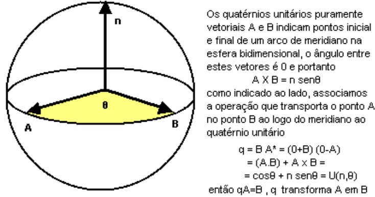
Figura 3.6: Vetor Esférico.
