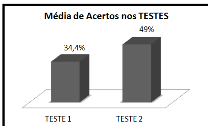
Figura 4.3: Gráfico da Média de Acertos
