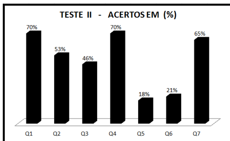
Figura 4.2: Gráfico de acertos do TESTE II
