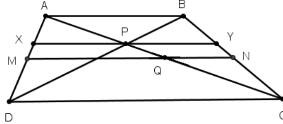
Figura 1.3: Trapézio ABCD
