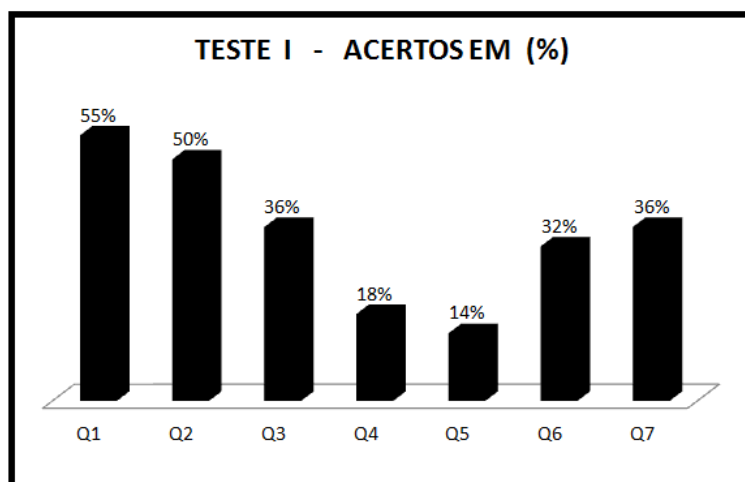
Figura 4.1: Gráfico de acertos do TESTE I
