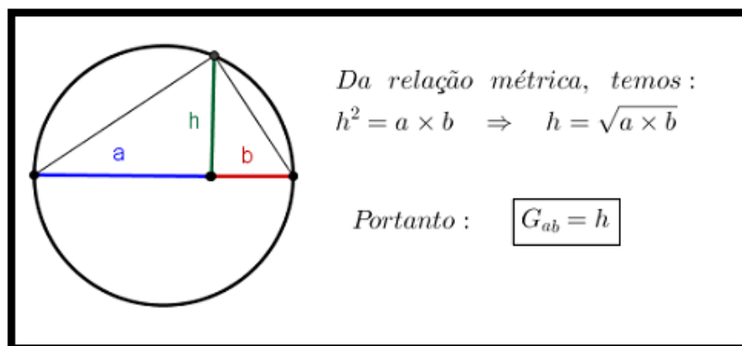
Figura 1.7: Representação da Média Geométrica
