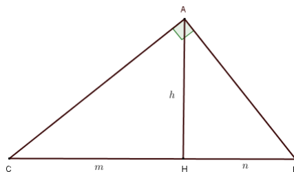
Figura 1.1: A altura é a Média Geométrica das projeções dos catetos sobre a hipotenusa.
