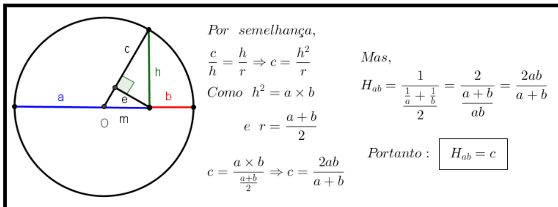
Figura 1.8: Representação da Média Harmônica
