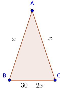
Figura 4.1: O triângulo isósceles do enunciado
