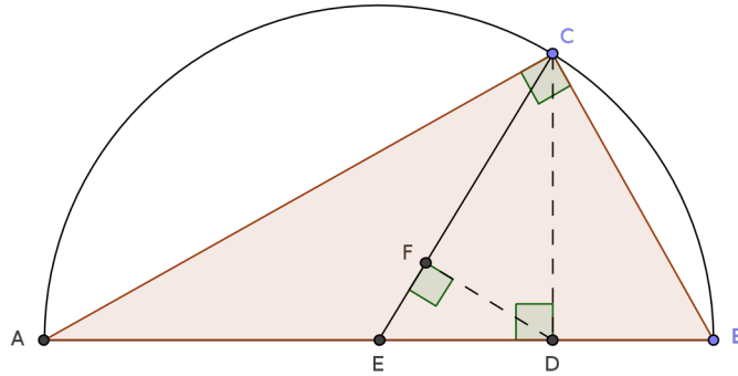
Figura 5.1: Triângulo ABC inscrito na semicircunferência
