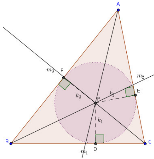
Figura 4.4: Incentro do triângulo ABC
