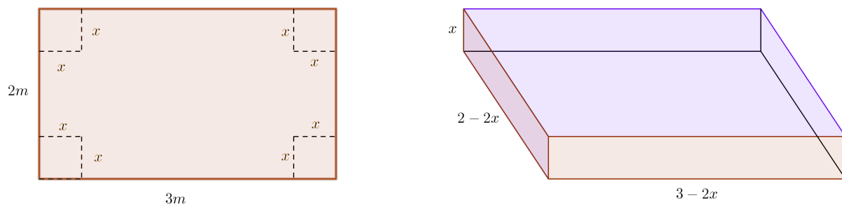
Figura 4.6: Cartolina demarcada e caixa aberta montada
