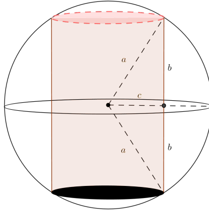
Figura 4.5: Configuração do enunciado que destaca o triângulo retângulo de lados a , b e c
