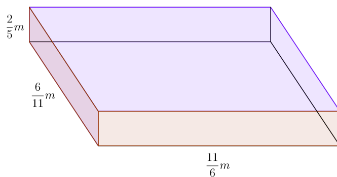
Figura 4.7: Representação das dimensões da caixa de volume máximo
