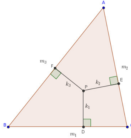
Figura 4.2: Uma configuração para o triângulo do enunciado
