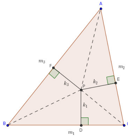
Figura 4.3: Os triângulos BPC , CPA e APB , destacados
