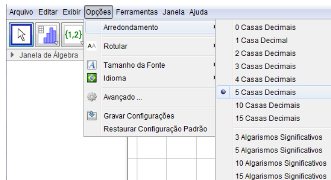
Figura 4.11: Arredondamento.
