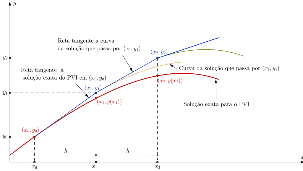
Figura 2.1: Método de Euler para determinar soluções próximas da solução exata do PVI (1.1)-(1.2).
