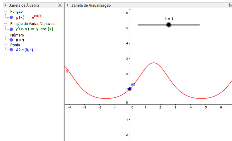
Figura 4.6: Solução exata.
