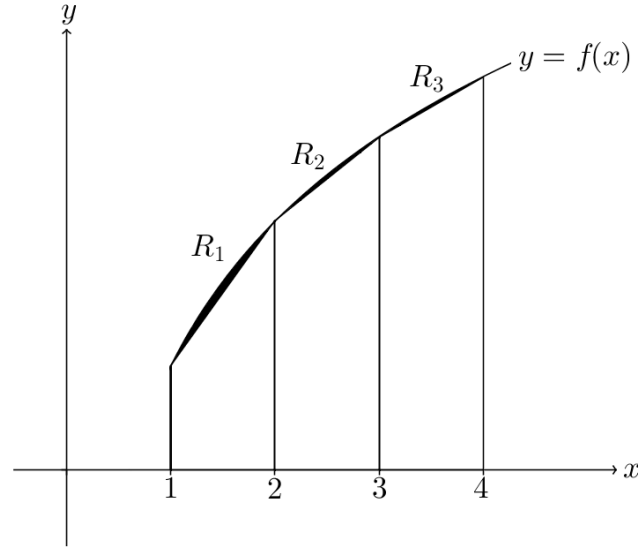
Figura 3.2: Interpretação geométrica do resultado da Proposição 3.6.
