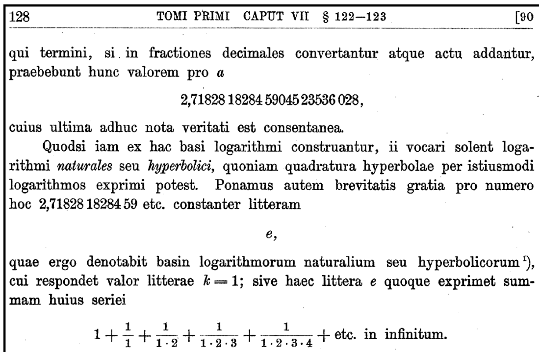
Figura 1.1: Trecho da obra Introductio in analysin infinitorum , de Leonhard Euler.
