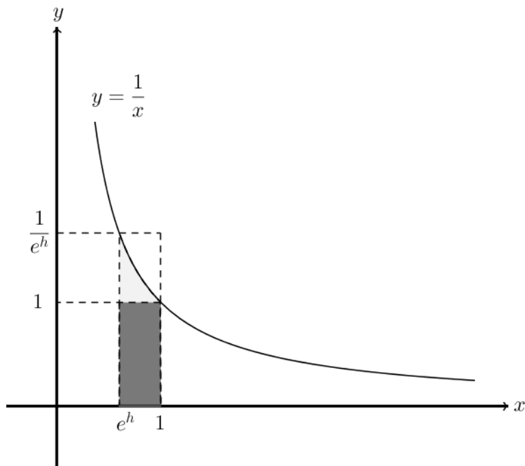
Figura 1.4: Representação da faixa da hipérbole H_1^{e^h} para h < 0 .
