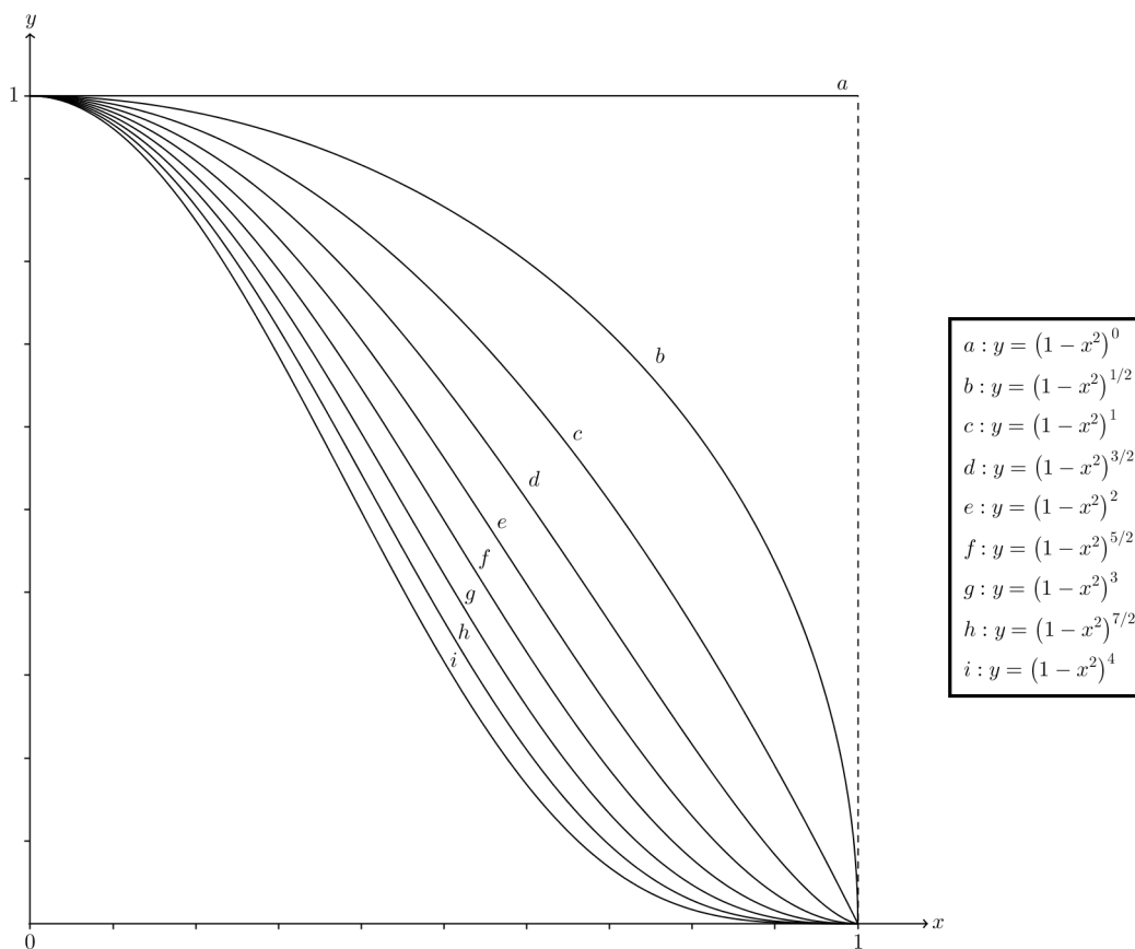
Figura 3.1: Gráfico de y = (1 - x^2)^n para n = 0, 1/2, 1, 3/2, 2, 5/2, 3, 7/2, 4 .
