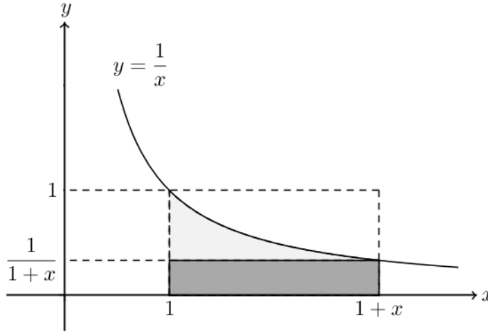
Figura 1.2: Representação da faixa da hipérbole H_1^{1+x} para estimativa de \ln(1+x) .
