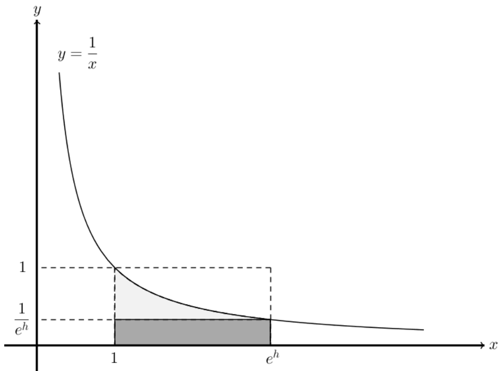
Figura 1.3: Representação da faixa da hipérbole H_1^{e^h} para h > 0 .
