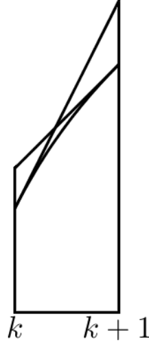
Figura 3.3: Trecho da curva y = f(x) limitado pelas retas x = k e x = k + 1 .
